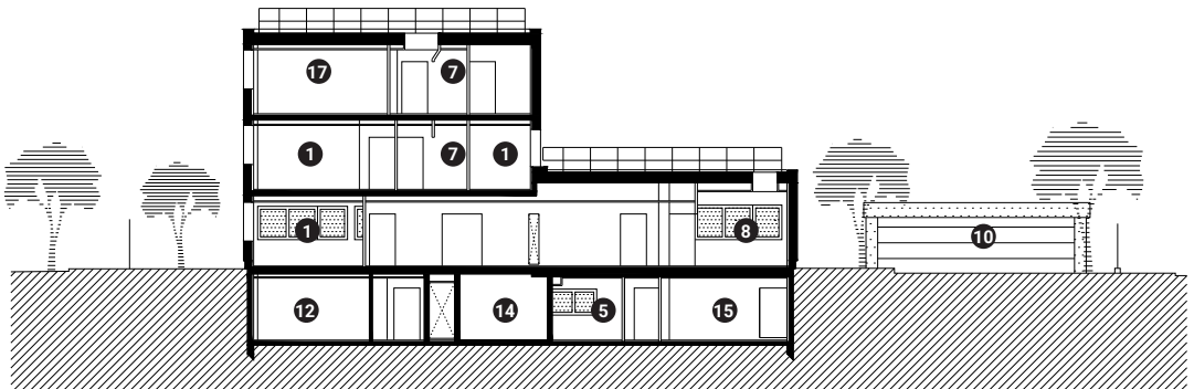
coupe longitudinale
